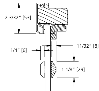
1 1/8" SDL (PUTTY LINE)
