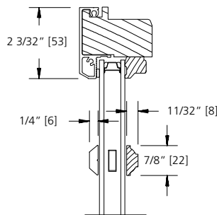
7/8" SDL BAR (PUTTY LINE)
