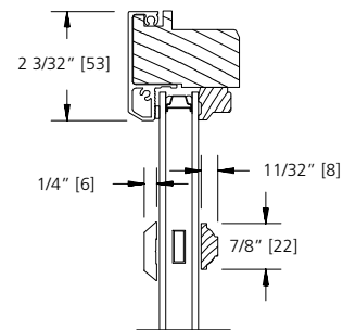
1 1/8" SDL BAR (PUTTY LINE)
