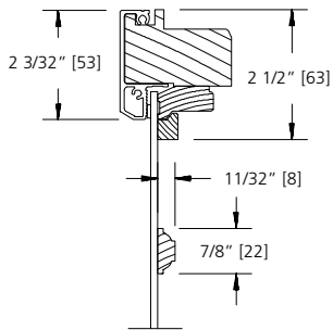
7/8" GRILLE BAR
