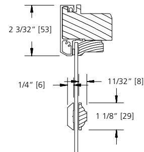
1 1/8" SDL (PUTTY LINE)
