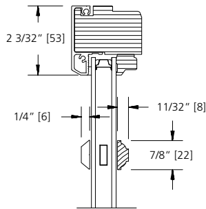
7/8" SDL BAR (PUTTY LINE)
