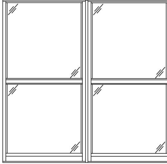
Twin Vent Max Size 107" x 72"
